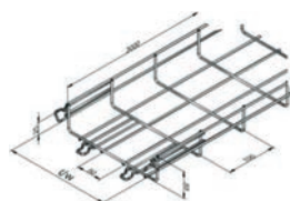
Chemin de câbles Fil CITO Chemin de câbles fil CITO, finition EZ, entièrement automatique, sans éclisses, ni boulons. S'assemble en un simple clic pour une résistance équivalente à un éclissage traditionnel, se monte en 5 secondes !
